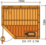
1616LAC INT. VOL. 3.77 m 3 MX 3.6 KW
